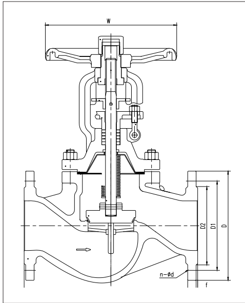
DN150
