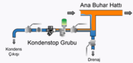
Buhar ve Kondens Tesisatında Bağlantı Şekilleri
