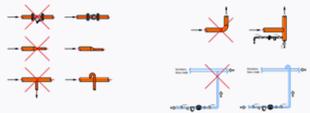
Buhar ve Kondens Tesisatında Bağlantı Şekilleri
